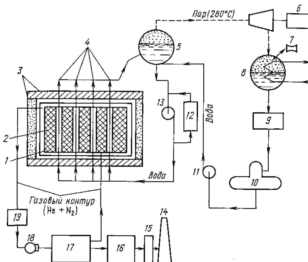
Рис. 11. Схема основных технологических контуров АЭС с реактором РБМК:
